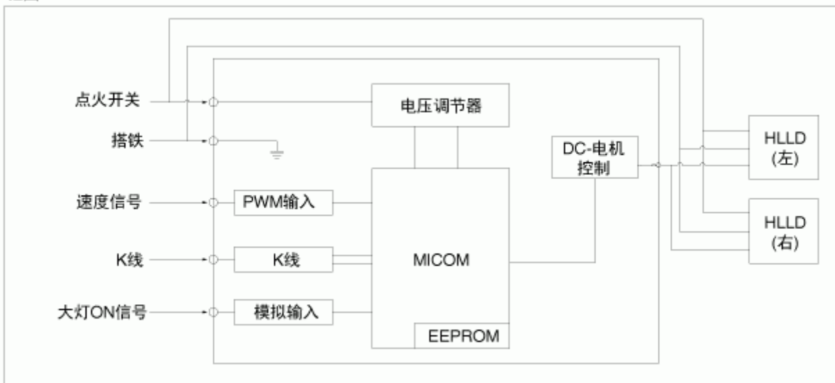
框图
